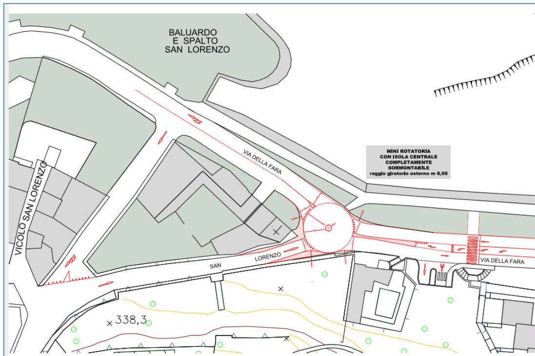
Fig.1 - Stralcio rappresentazione grafica della nuova rotatoria oggetto di intervento.
